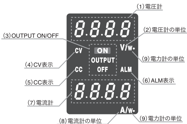
図 6-2 表示部
