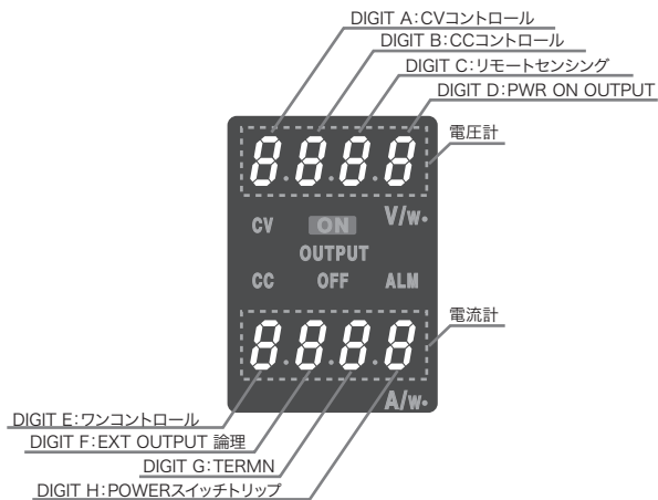
図 3-2 CONFIG 表示
